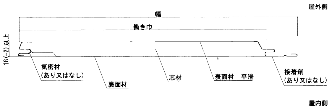
外装材断面
