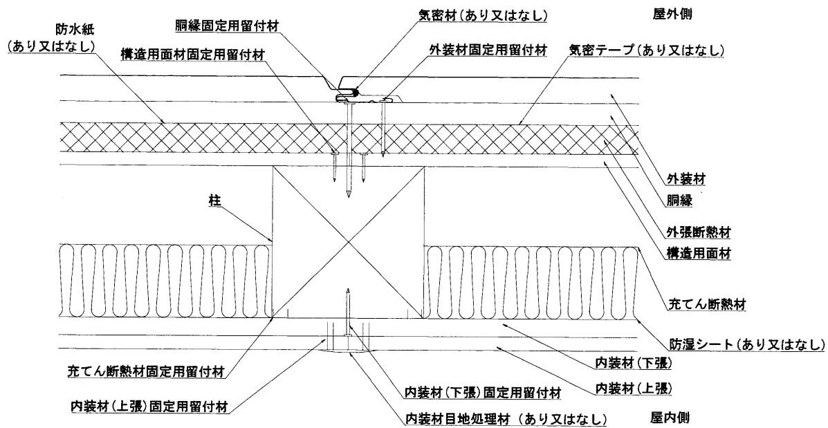
水平断面詳細図
