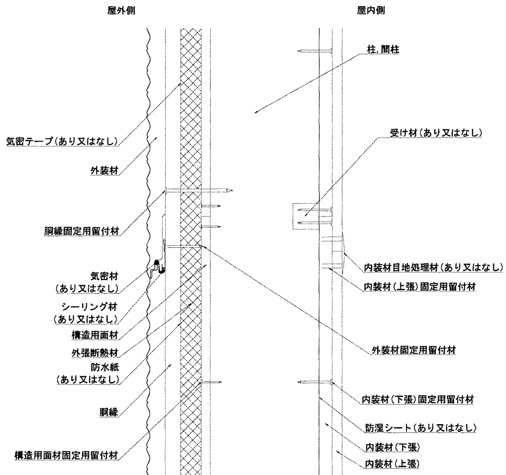
図2 構造説明図(充てん断熱材なし)
