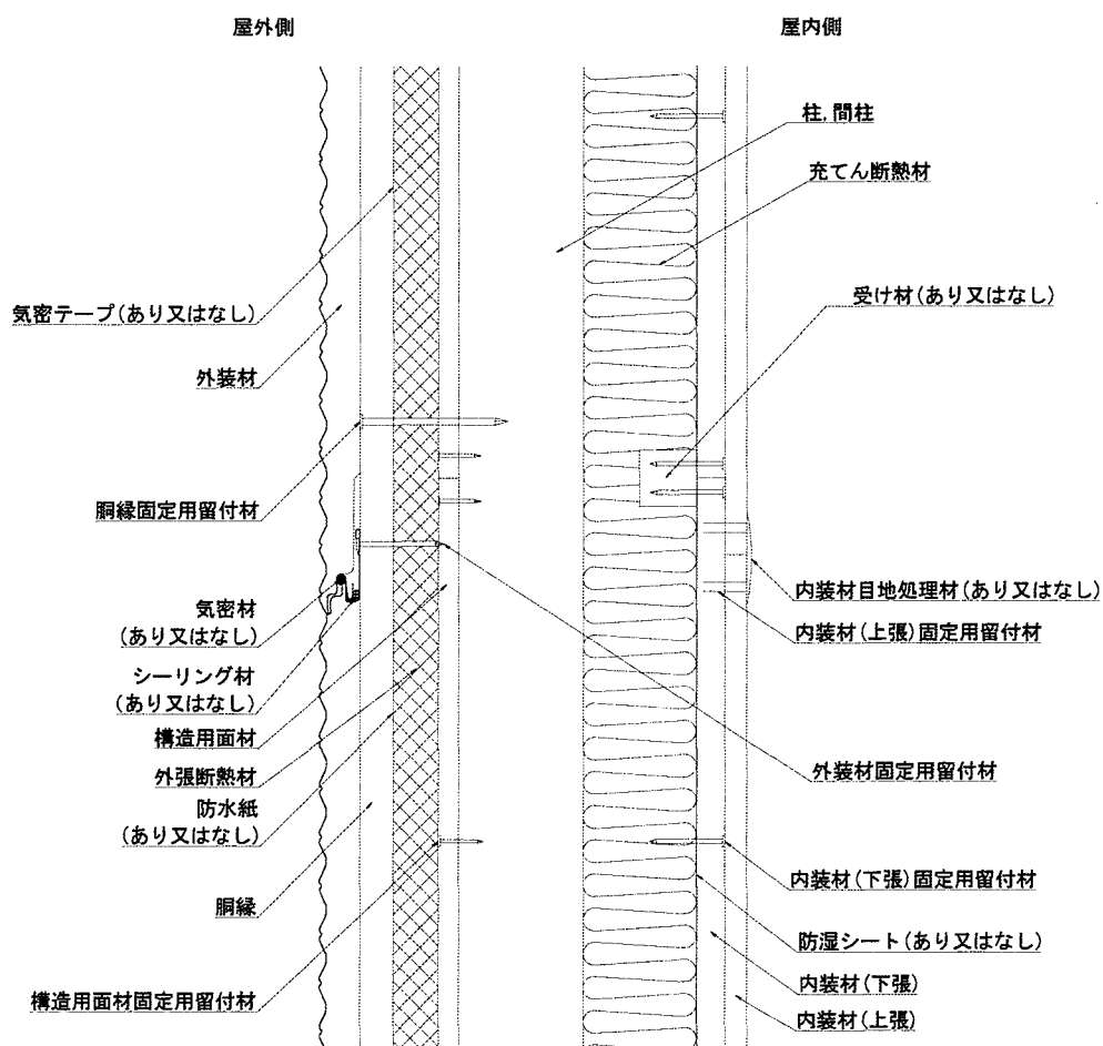
図2 構造説明図(充てん断熱材あり)
