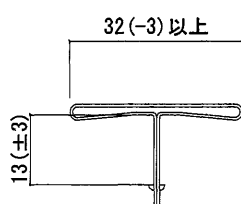
目地カバー(鋼板製) 1ピースタイプ
