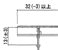
目地カバー(鋼板製) 2ピースタイプ
