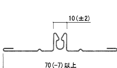
目地受け(鋼板製)
