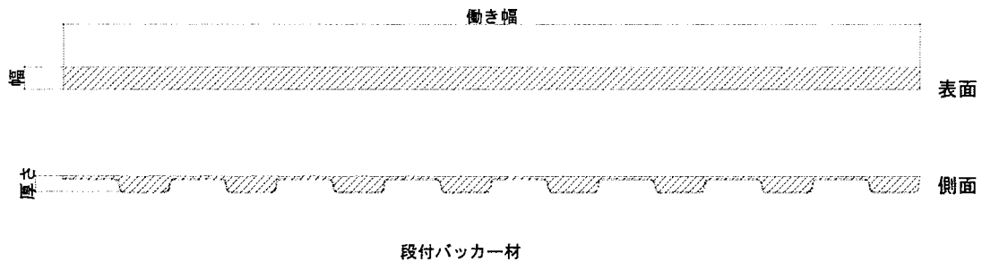
図3 構造説明図
