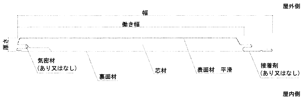
外装材断面
