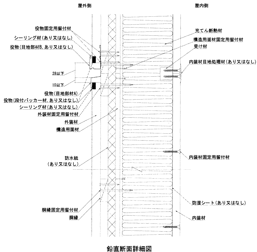
図2 構造説明図(内装材単張仕様)
