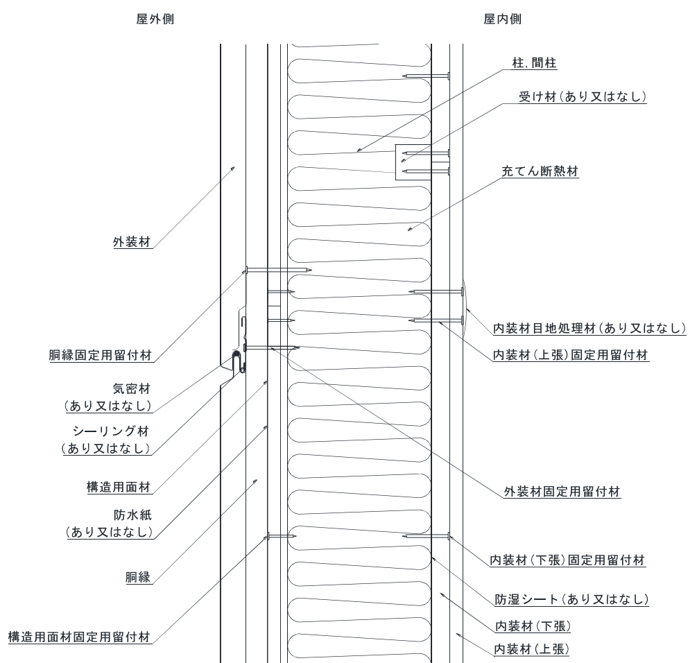
鉛直断面図
