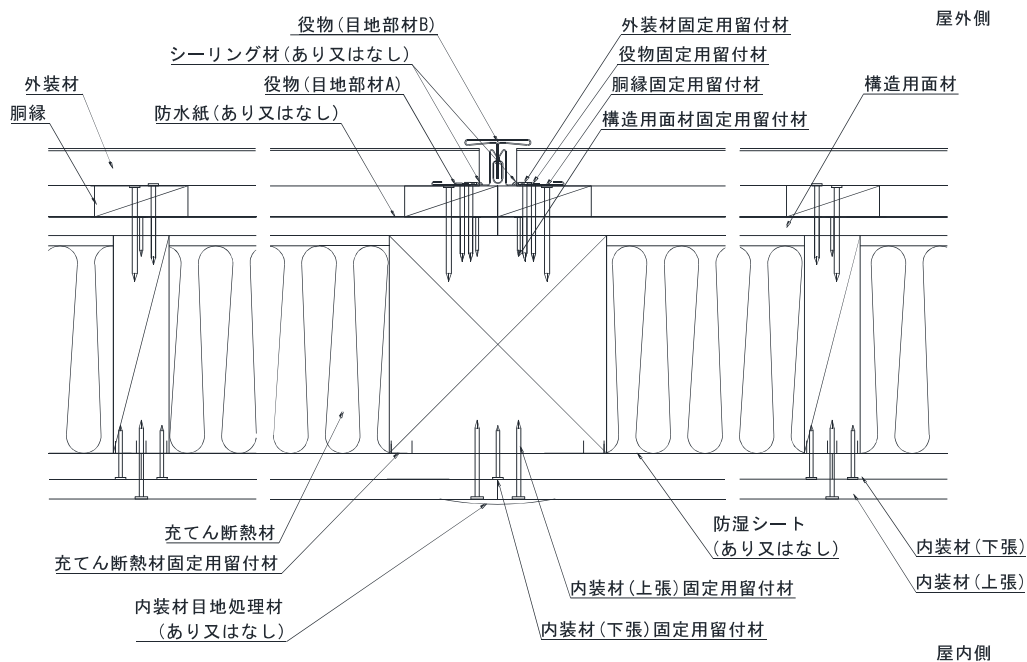
水平断面図
