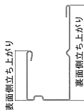
目地部材B 断面図(例)
