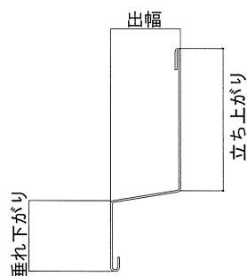
目地部材A 断面図(例)
