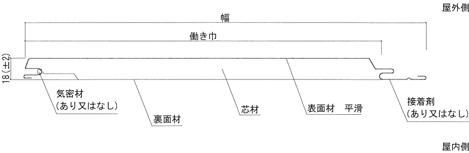
外装材断面
