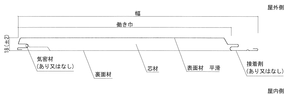
外装材断面
