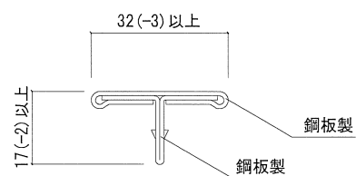
目地部材B(2ピースタイプ)
