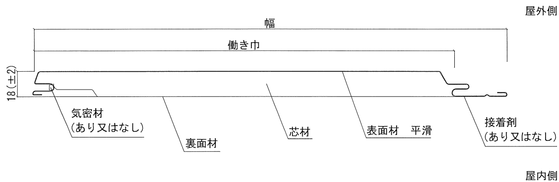
外装材断面
