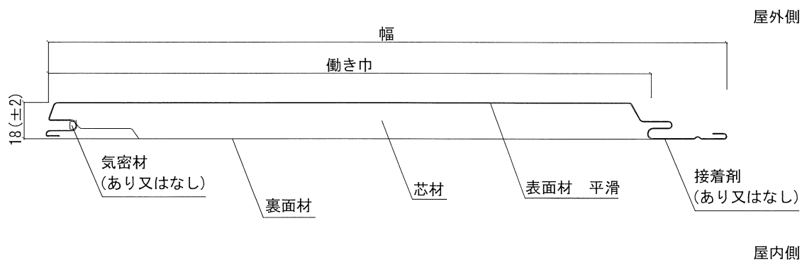
外装材断面
