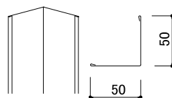
入隅50 (JR1900)
