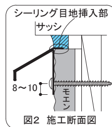
図2 施工断面図
