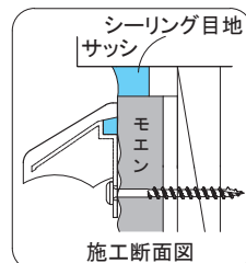
施工断面図
