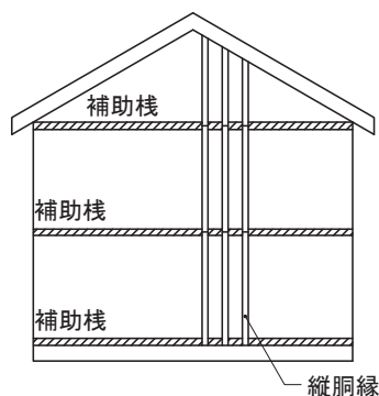
妻側の壁
