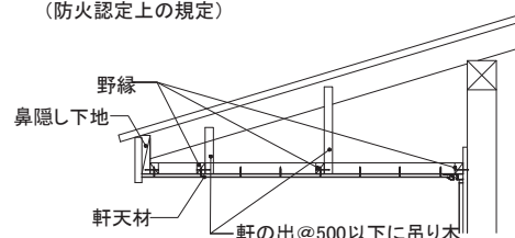
軒の出が500～2000mm以下の場合
