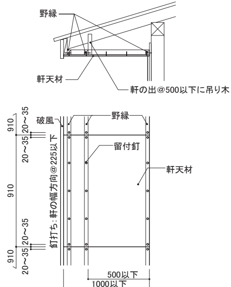
軒の出が500~1000mm以下の場合
