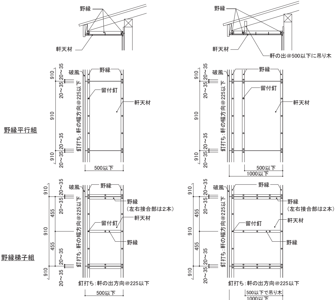
軒の出が500mm以下の場合
