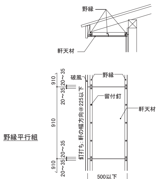
軒の出が500mm以下の場合
