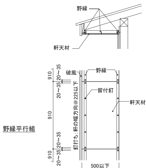
軒の出が500mm以下の場合
