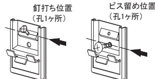
<留付金具EX出隅用II: JE652C・JE552C>
