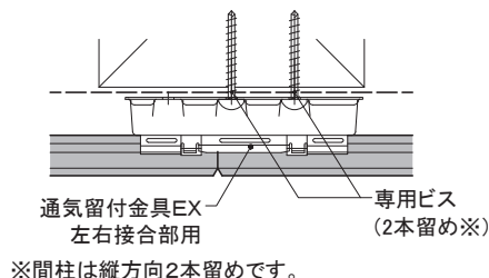
※間柱は縦方向2本留めです。
