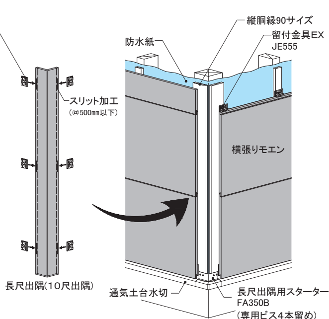
図2 モエン本体横張り
