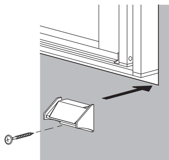
＜雨跡防止水切：ピースタイプ＞
