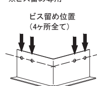
<長尺出隅用スターター: FA350B> ※ビス留め専用
