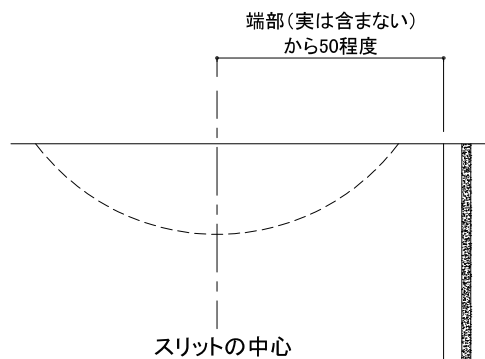
図10 端部のスリット加工位置
