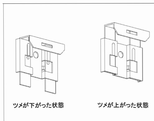
図5 スリット加工部用留付金具Ⅱ
