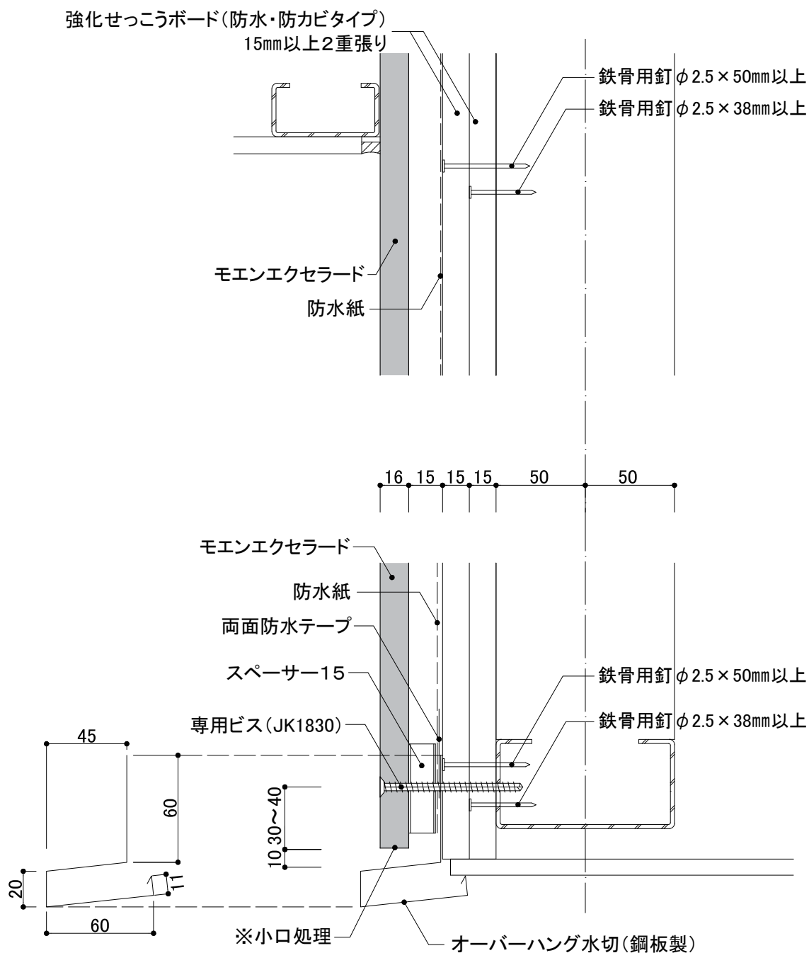
断面詳細図
