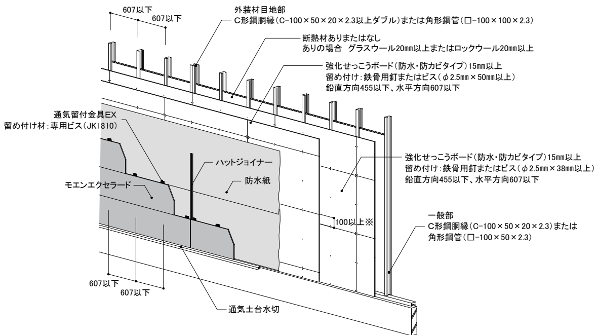
下地組図(屋外側)
